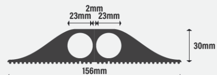
TYPE FF Zwart / Noir 4,5m C414.01
