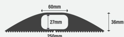
TYPE H Zwart / Noir 1,5m C441.01
