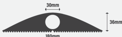
TYPE G Zwart / Noir 4,5m C434.01
