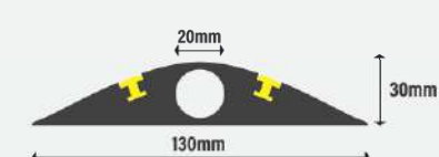
TYPE TTC/1 Zwart-Geel / Noir-Jaune 4,5m C504.01
