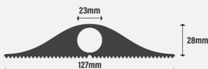
TYPE F Zwart / Noir 4,5m C404.01 9m C409.01
